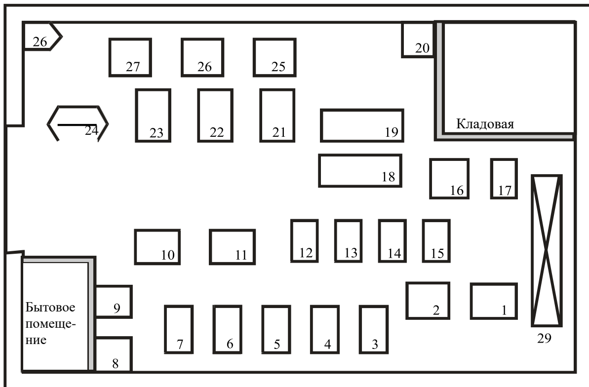
Вариант В План механического цеха
